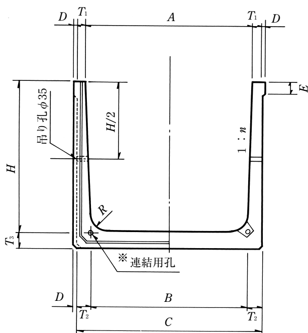
断面図
