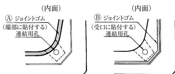
製品接合部
