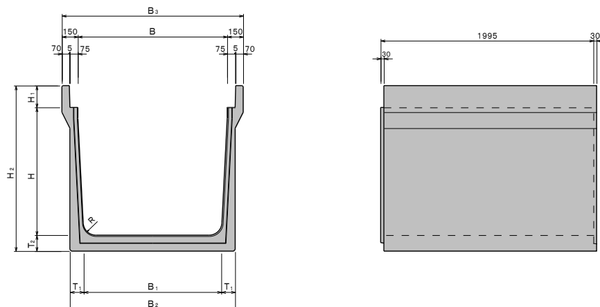
形状図
