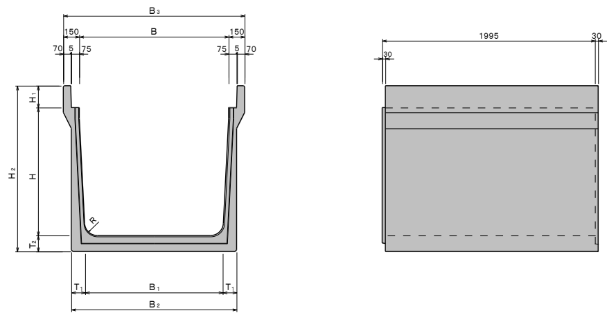
形状図
