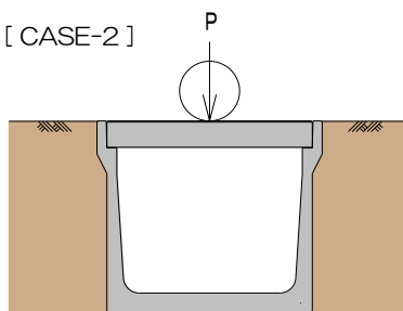
標準断面図
