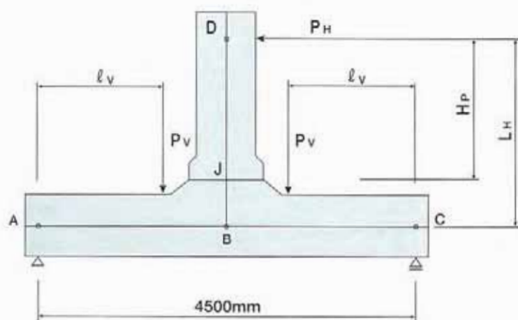
載荷位置図
