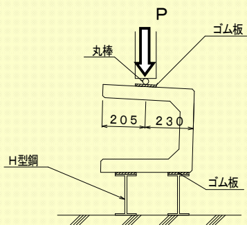
高強度集水フリューム
